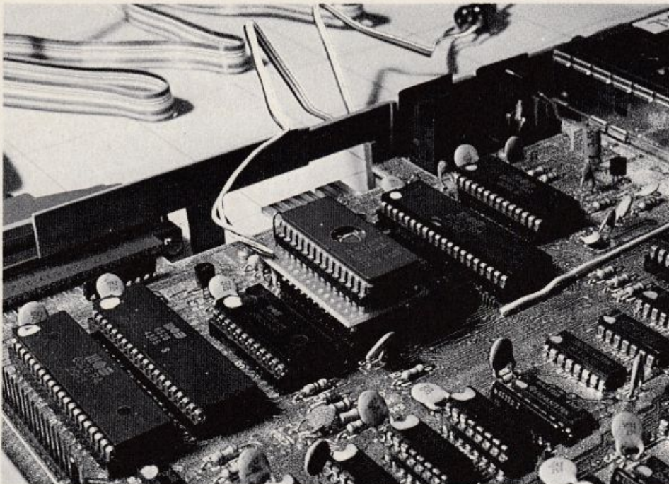
Figura 2. Eprom dello SpeedDOS installata sul C64.
